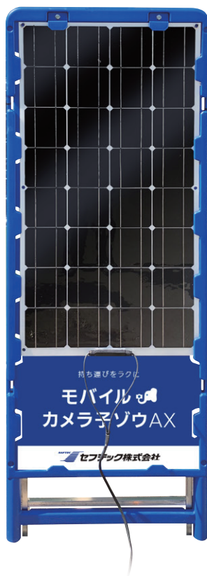
■看板付きソーラーパネル仕様 100W 単結晶シリコンパネル
